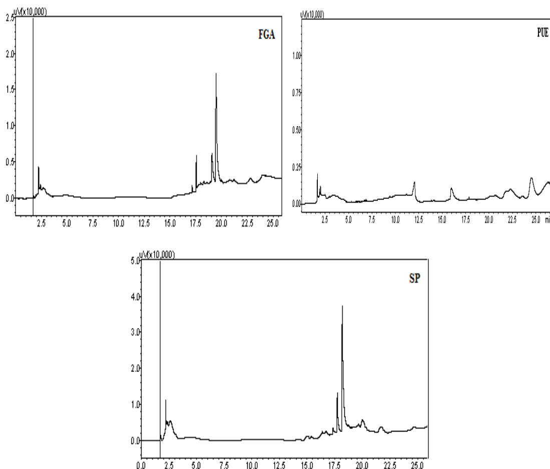
Figura 2. Cromatogramas demonstrando a presença de ácidos orgânicos na parte aérea de leguminosas utilizadas como adubação verde no Agreste Pernambucano. Ve+E= Vegetação espontânea+esterco, CAL= Calopogônio, EST=Estilosantes, CRO= Crotalária, FGA= Feijão Guandu Anão, PUE= Puerária e SP= Soja Perene. (1) Propiônico (2) Butírico (3) Acético (4) Shiquímico (5) Isobutírico.
