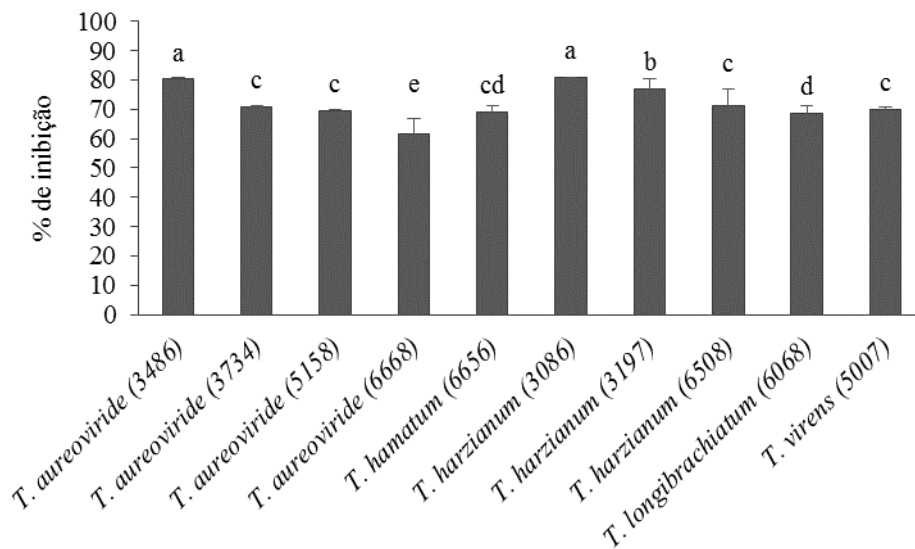
Figura 4. Efeito antagonista de isolados de Trichoderma contra o crescimento micelial de Scytalidium lignicola (CFF408), in vitro . Médias seguidas pela mesma letra não diferem estatisticamente entre si pelo teste de Tukey ( P \leq 0,05 ).
